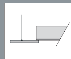
Installazione ad incasso False ceiling recessed installation
